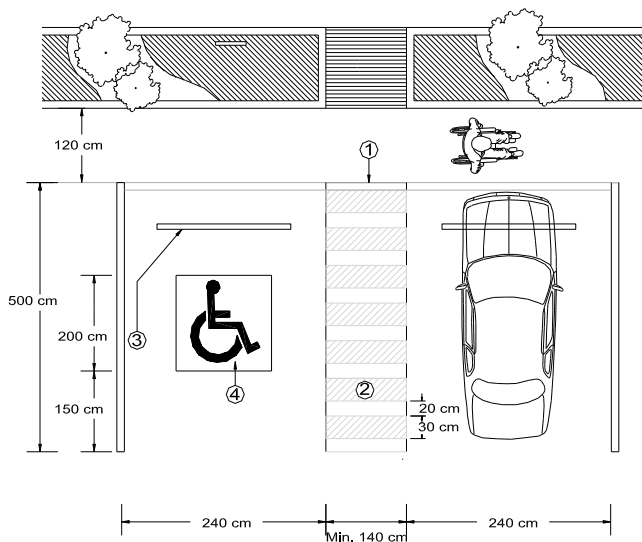
Planta
