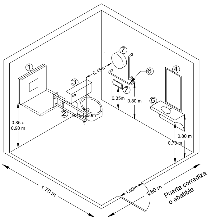
Isométrico
